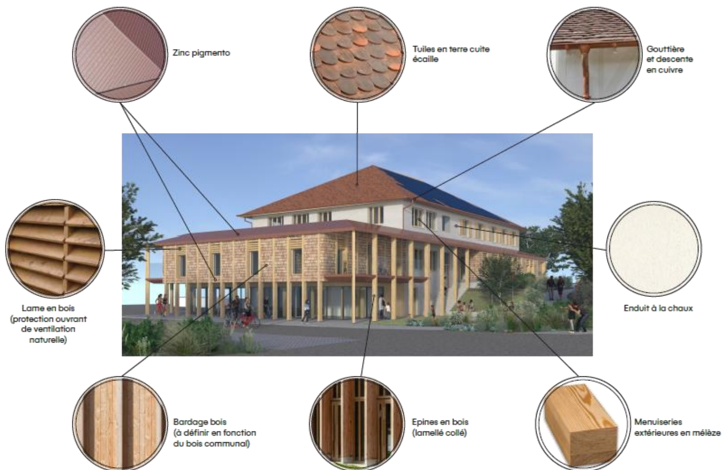
Matériaux façade
